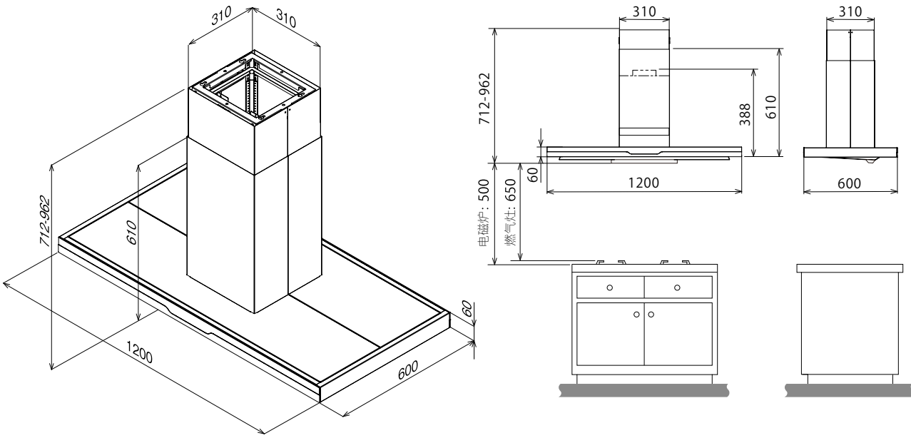
尺寸图 [mm]
