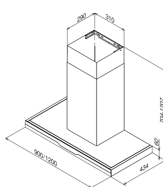
尺寸图 [mm]
