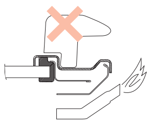
进风不足火焰呈黄色
