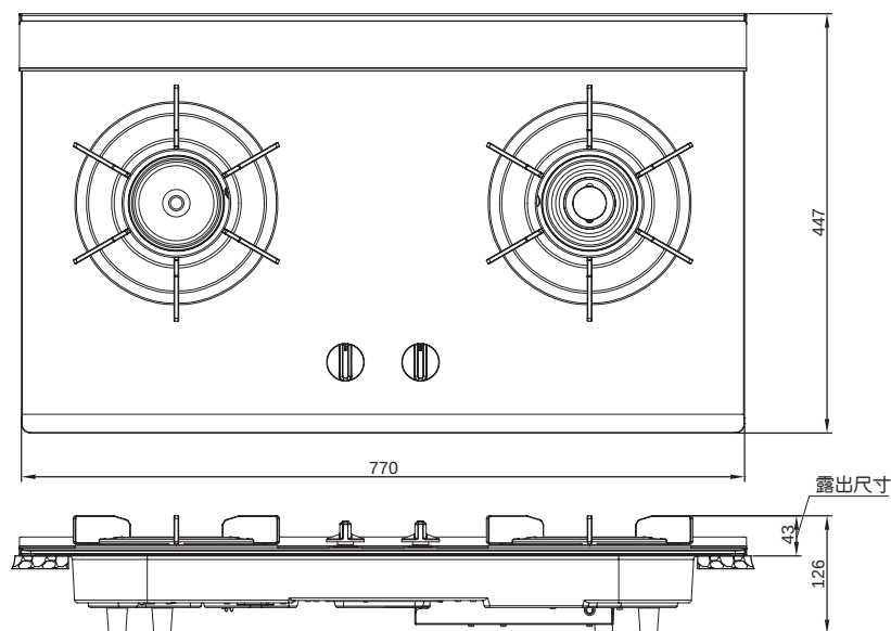
外形尺寸
