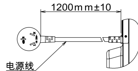
Detail:A(Scale1:5)
